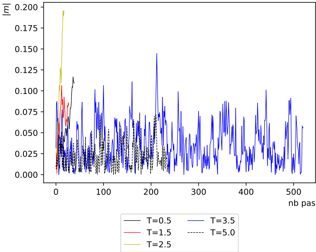
Evolution de l'aimantation sur critère \pm 5\% de la moyenne, N=64
